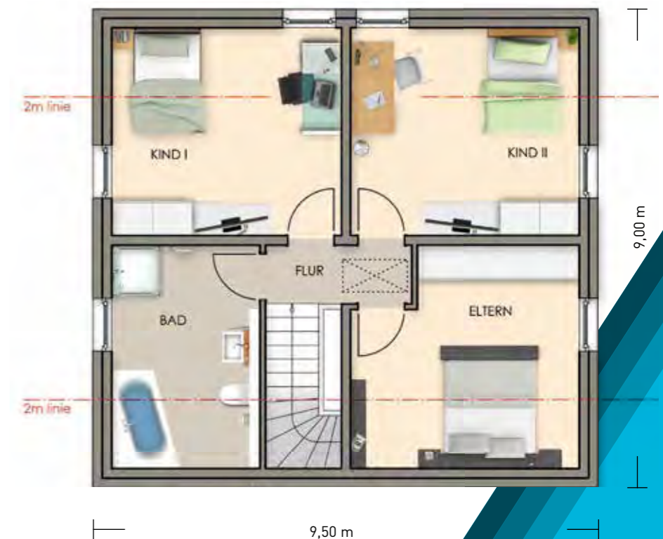
1:100 Dachgeschoss
