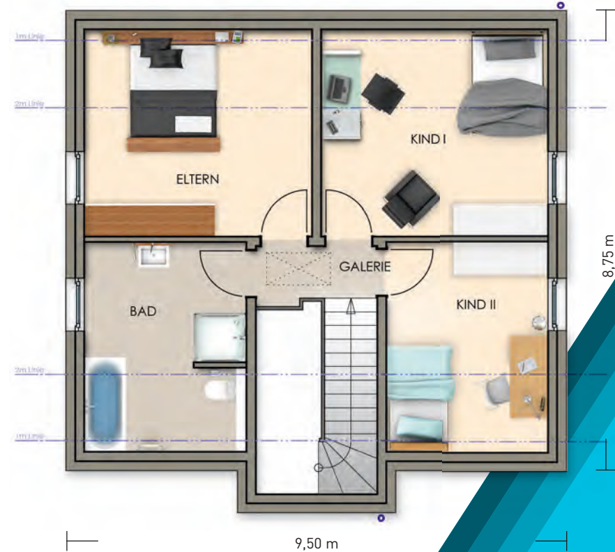
1:100 Dachgeschoss
