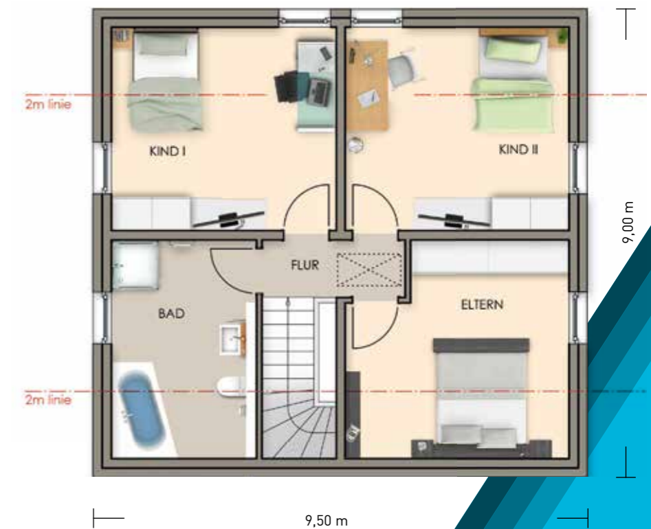
1:100 Dachgeschoss
