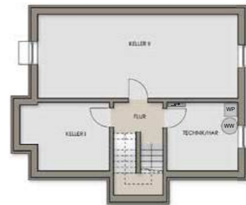
Untergeschoss (optional) Darstellung verkleinert
